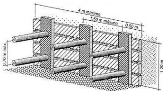
Exemple d'estrebació horitzontal
